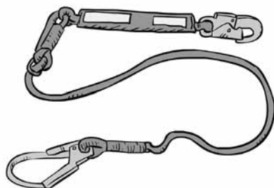
Figura 1. Ejemplo de absorbedor de energía incorporado al elemento de amarre.
