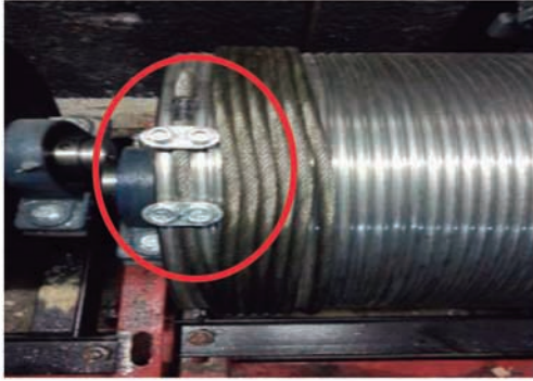
La grapa de amarre del tambor de arrollamiento expulsa el cable del canal
