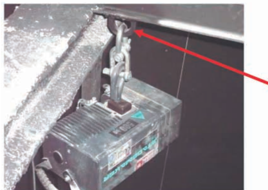
Los elementos portantes de los equipos deben ser verificados (por ejemplo, los cáncamos soldados)
