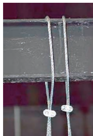
Las mordazas (perrillos) en las eslingas no están permitidas como elementos de elevación de cargas
