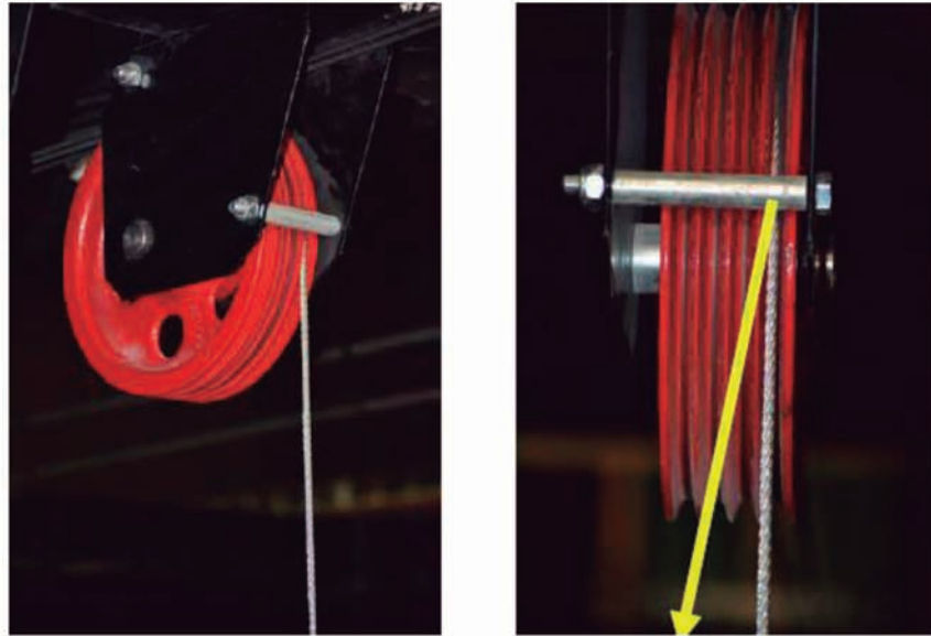
Ángulo de desvío en poleas, excesivo en el montaje de concha acústica
