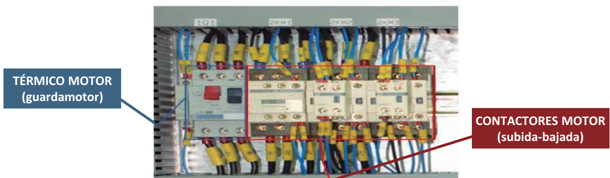
Identificación de algunos componentes del cuadro elevador de foso
