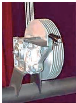
Cabrestante y poleas de cabeza fijadas a la estructura con soldadura
