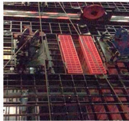
Peine protegido con tramex
