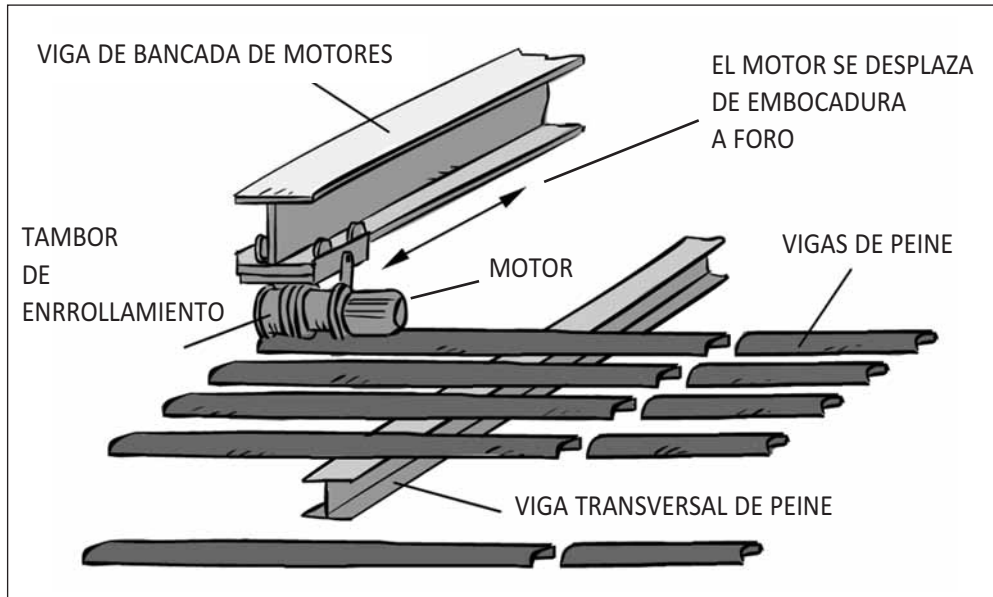
Detalle de la instalación de un motor de velocidad variable o fija (tiro contrapesado y motriz)
