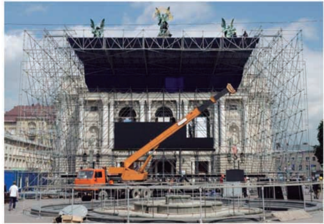
El uso de equipos específicos para trabajos en altura, evita el empleo de otros equipos no diseñados para esta tarea
