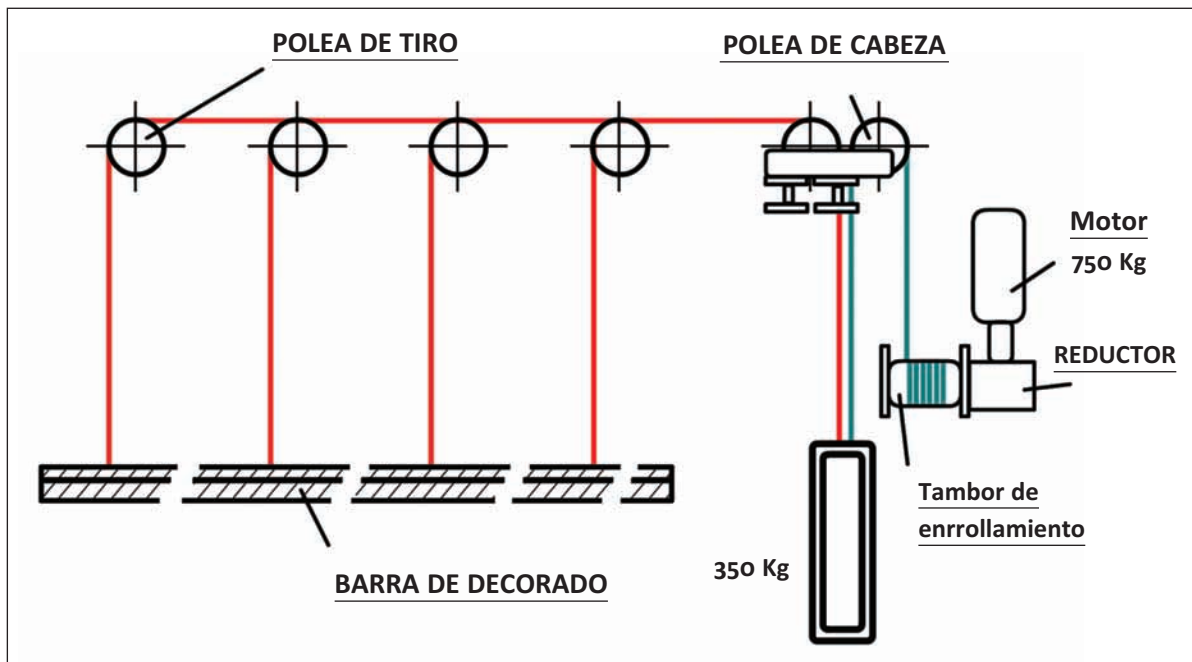
Esquema habitual de tiro contrapesado y motorizado (motor con sistema de control por mesa y etapas de potencia de velocidad variable)
