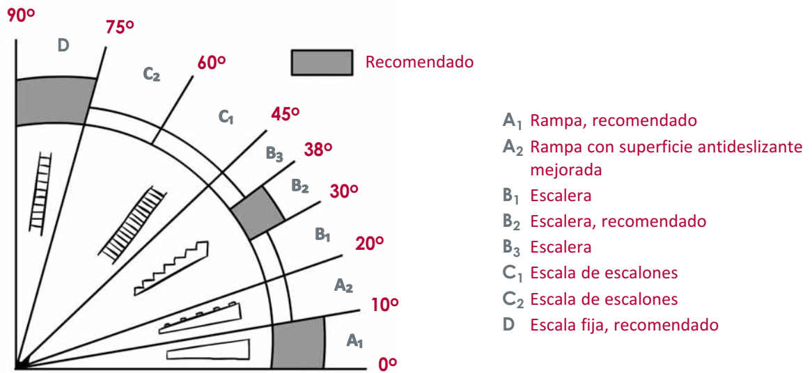
Gama de los diferentes medios de acceso
